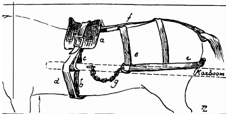
AFB. IV a. zaal of kussen , b. kussenriem , c. licht of help , d. kwikriem , e. broek , f. achterreep , g. deinskeet .
