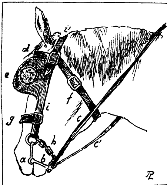
AFB. II HOOFDSTEL of Breil . a. gebit , b. brank , c. c' loenie , d. kopstuk , e. ooglap , f. keelband , g. neusriem , h. kinnekeet , i. i'. portemors .
