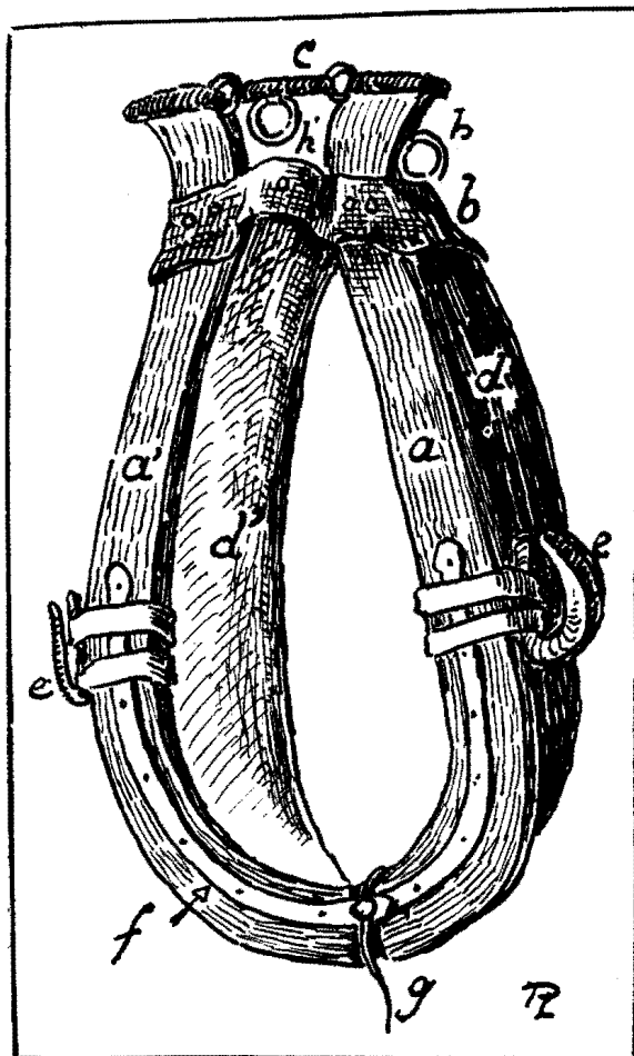
AFB. I. GAREEL. a-a'. spaan. b. kap. c. spanriem, d: goreelbulg , d': goreelkussen , e-e'. treit , met treithuak en treitkussen , f. spaan-ijzer , g. goreelgesp , h-h'. ogen .
