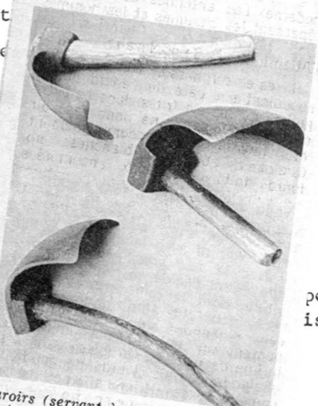
De bas en haut : compas bourguignon du XVIII e siècle, compas compagnonique, compas girondin.
